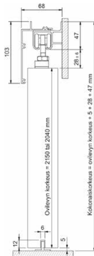
Slide 2100 ja 3000 leikkauskuva
