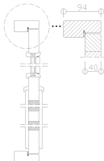
Rakennekuva mökkiovesta.
