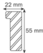
WC kynnys M7-M9
