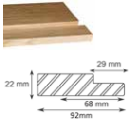
92/29 kyntteellinen M7-M10 M12,13,15,17 68/29 kyntteellinen M7-M10
